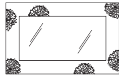
M 305 specchiera mirror cm 144xh90
