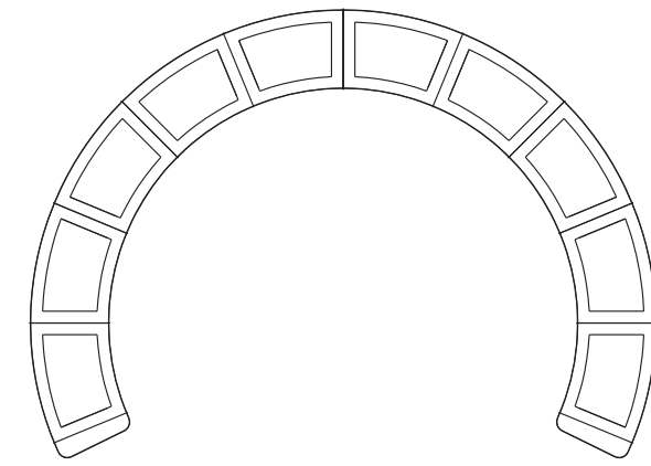
Tavolo riunione Meeting table cm 645 x 462 h 76
